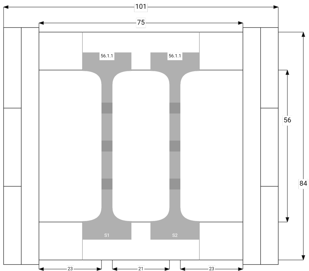
Die Bemaßung der Innenaufteilung wird gerundet dargestellt. Einheit: mm / The interior separation dimension shown is rounded. Unit: mm
